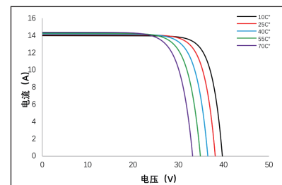
电流-电压曲线 BM8S-T54HD-420
