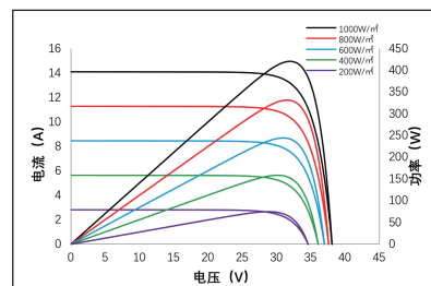
电流/功率-电压曲线 BM8S-T54HD-420
