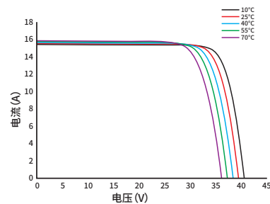
电流-电压曲线 BM9R-T54HDB-490
