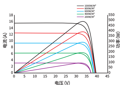
电流/功率-电压曲线 BM9R-T54HDB-490
